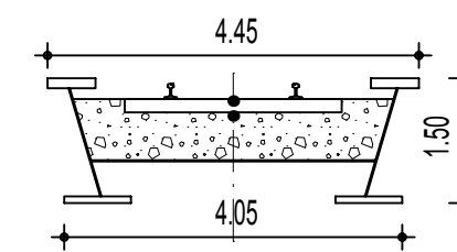
Brückenquerschnitt Stahltrug M 1:100
