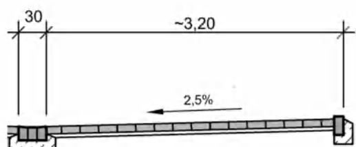
Mischfläche
